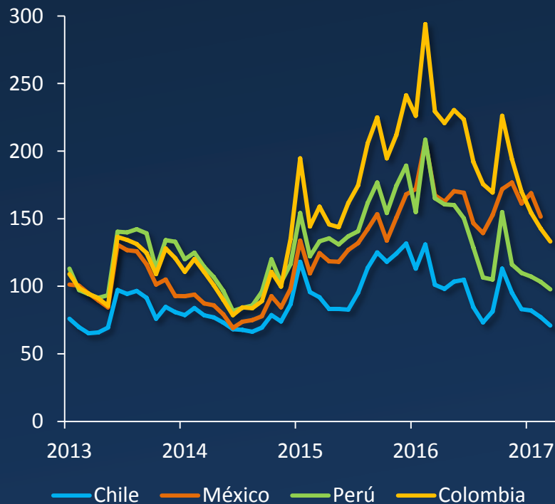
CDS países Alianza del Pacífico (Puntos base)
